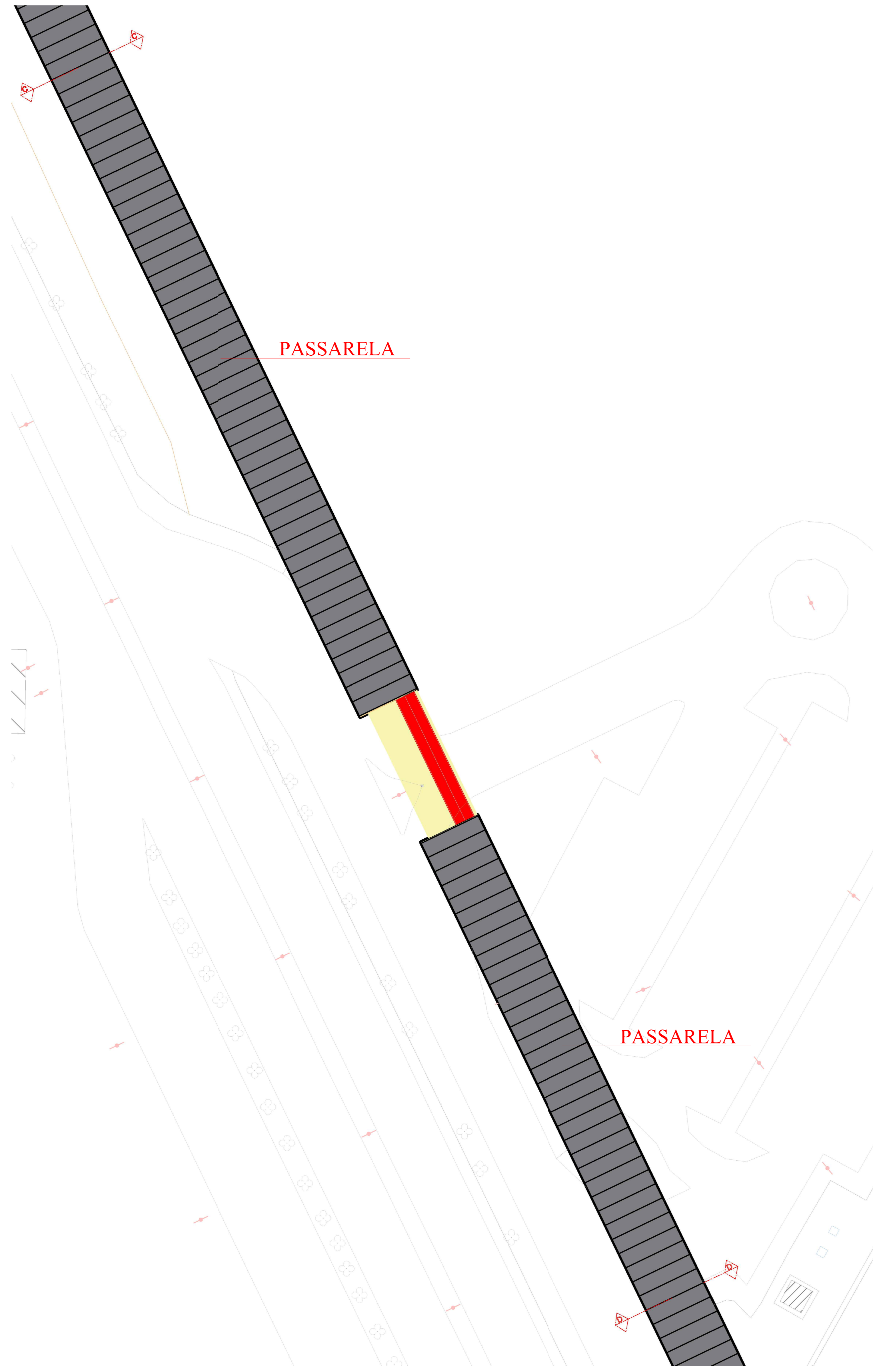
④ PLANTA DE LOCAÇÃO PASSARELA Esc. 1:250
